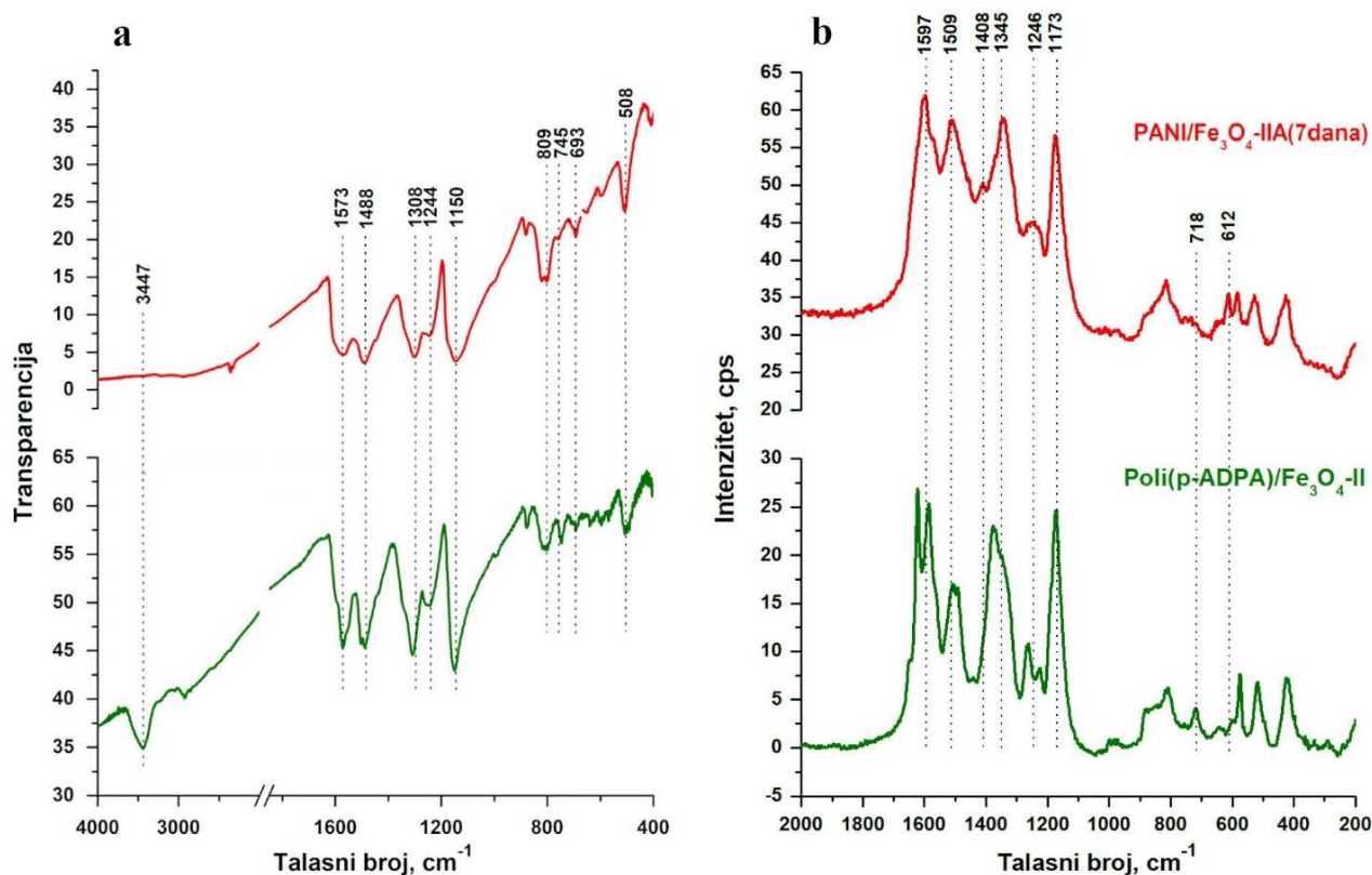
Slika 4.44. FTIR (a) i ramanski spektri (b) uzoraka PANI/Fe 3 O 4 -IIA(7) i Poli(p-ADPA)/Fe 3 O 4 -II.
