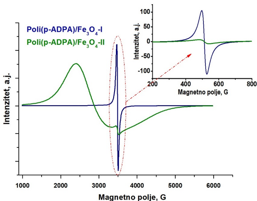
Slika 4.41. EPR spektri uzoraka Poli(p-ADPA)/Fe 3 O 4 -I i Poli(p-ADPA)/Fe 3 O 4 -II u oblasti 5000 G (na insetu je prikazan EPR signal sa korigovanom baznom linijom u oblasti 600 G).
