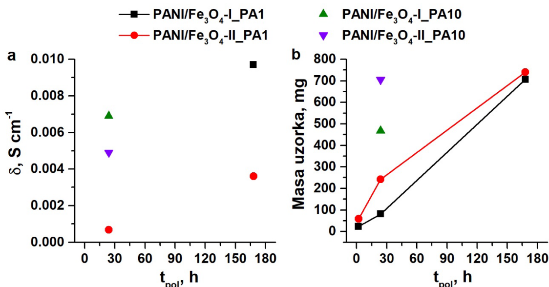
Slika 4.31. Uticaj uslova sinteze (koncentracije p-ADPA, t_{\text{pol}} i m(\text{Fe}_3\text{O}_4)/m(\text{ani}) ) na električnu provodljivost (a) i masu uzorka (b).
