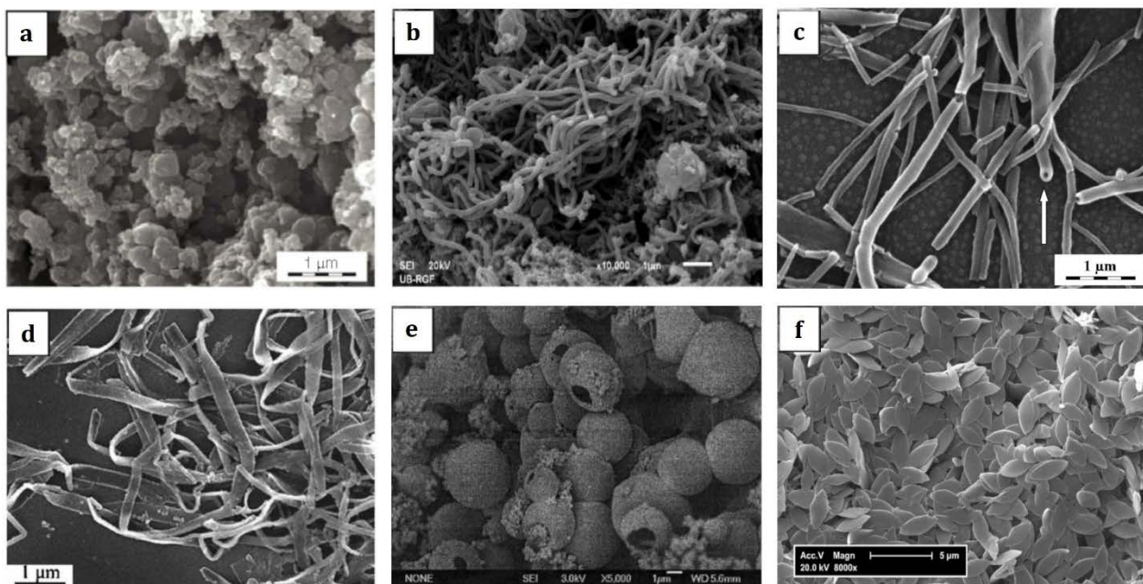
Slika 1.19. SEM mikrofografije nekih supramolekulskih struktura PANI: a) granule; b) nanovlakna; c) nanotube; d) nanotrake; e) šuplje mikrosfere i f) nanolistići. Slike preuzete i adaptirane sa dozvolom iz referenci [137,138,143–146].
