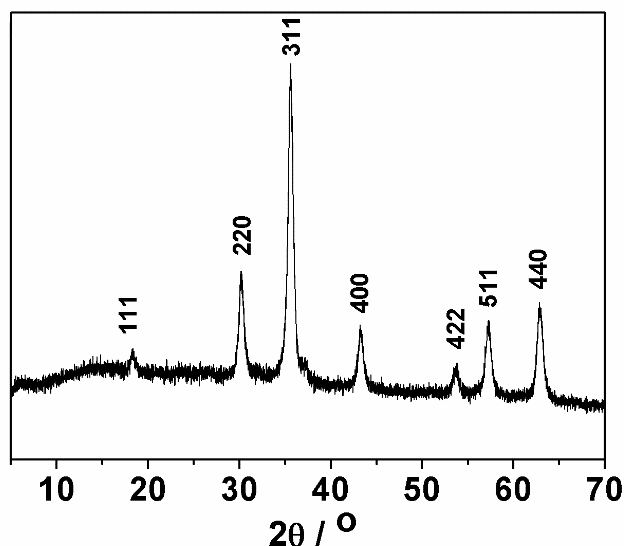
Slika 4.2. Difraktogram praha sintetisanih nanočestica \text{Fe}_3\text{O}_4 .
