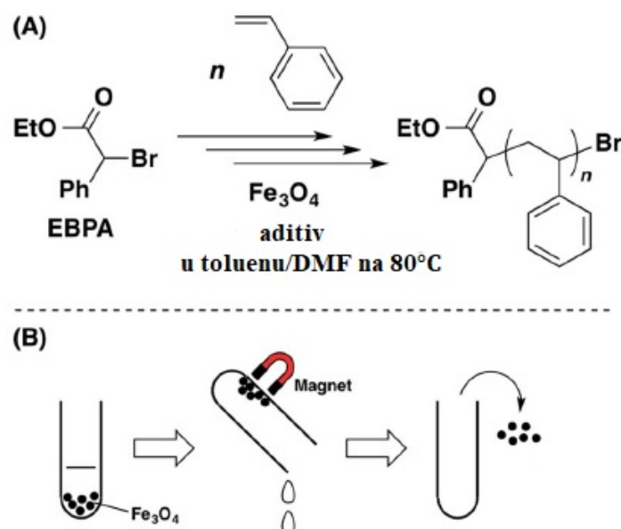
Slika 1.8. A) Radikalna polimerizacija stirena upotrebom nanočestica \text{Fe}_3\text{O}_4 i B) izdvajanje nanočestica \text{Fe}_3\text{O}_4 nakon reakcije polimerizacije. Slika preuzeta i adaptirana sa dozvolom iz RSC Advances, Controlled radical polymerization of styrene with magnetic iron oxides prepared through hydrothermal, bioinspired, and bacterial processes, autora A. Kanazawa, K. Satoh, S. Kanaoka, M. Kakihana, M. Kobayashi, J. Sato, H. Imai, Y. Oaki, A. Arakaki, K. Katagiri, M. Kamigaito, S. Aoshima, 5, 51122-51129. Copyright (2015) The Royal Society of Chemistry.
