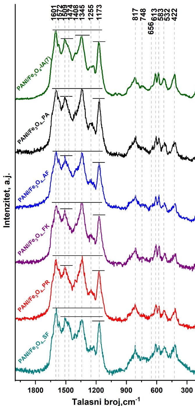
Slika 4.26. Ramanski spektri produkata oksidacije anilina sa \text{H}_2\text{O}_2 /APS u prisustvu različitih arilamina.
