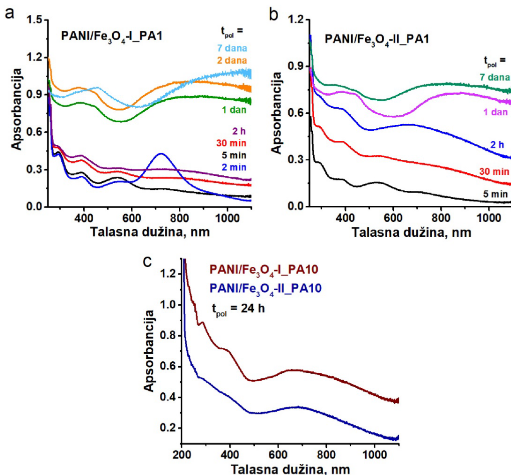
Slika 4.30. UV-Vis-NIR spektri suspenzija reakcionih smeša snimjeni tokom oksidacije anilina u prisustvu p-ADPA. Uoči merenja suspenzije PANI/Fe 3 O 4 -I_PA1 i PANI/Fe 3 O 4 -II_PA1 (a i b) su razblažene u vodi 10 puta, dok su suspenzije PANI/Fe 3 O 4 -I_PA10 i PANI/Fe 3 O 4 -II_PA10 (c) razblažene 45 puta.
