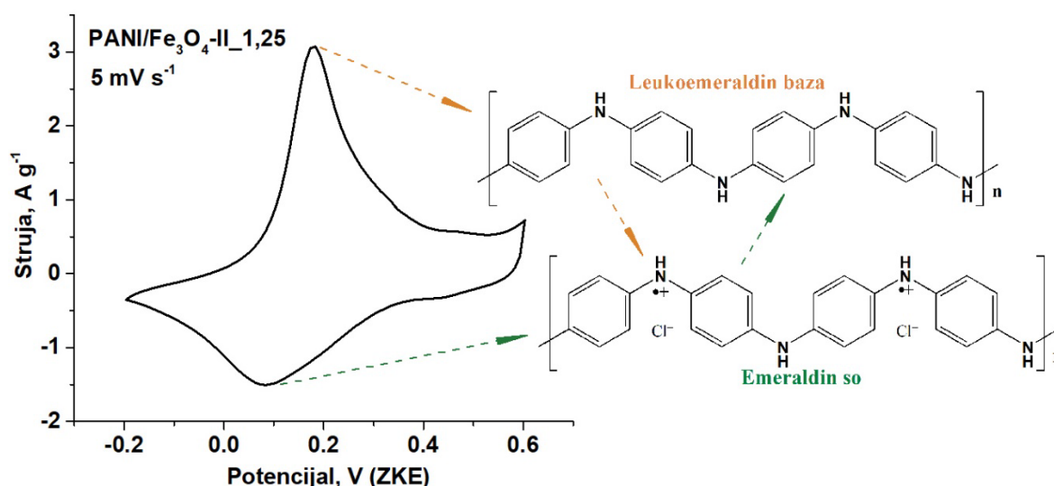
Slika 4.9. Ciklični voltamogram PANI/Fe 3 O 4 -II_1,25 snimljen u 1 M HCl pri brzini polarizacije 5 mV·s -1 u opsegu potencijala od -0,2 V do 0,6 V u odnosu na ZKE.
