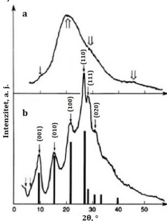
Slika 1.18. Difraktogrami a) PANI-EB (široke strelice pokazuju položaje maksimuma amorfne oblasti, a tanka strelica pokazuje refleksiju koja je najverovatnije posledica tragova ES) i b) PANI-ES (sa obeleženim kristalografskim ravnima). Slika preuzeta i adaptirana sa dozvolom iz Macromolecules, X-ray Structure of Polyaniline , autora J. Pouget, M. E. Józefowicz, A. J. Epstein, X. Tang, A. G. MacDiarmid, 24, 779-789. Copyright (1991) American Chemical Society.
