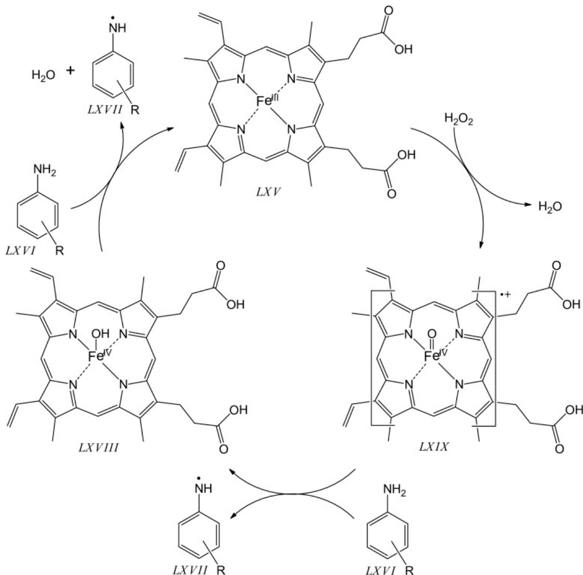
Slika 1.20. Ciklus peroksidaze za anilin ( \text{LXVI} , \text{R} = \text{H} ) i supstituisane aniline ( \text{LXVI} ). Hem B ( \text{LXV} ), supstituisani anilin radikal ( \text{LXVII} ), intermedijer II ( \text{LXVIII} ), intermedijer I ( \text{LXIX} ). Slika preuzeta i adaptirana sa dozvolom iz Chemical Papers, Enzymatic oligomerization and polymerization of arylamines: State of the art and perspectives, autora G. Ćirić-Marjanović, M. Milojević-Rakić, A. Janošević-Ležaić, S. Luginbühl, P. Walde, 71, 199-242. Copyright (2017) Springer.
