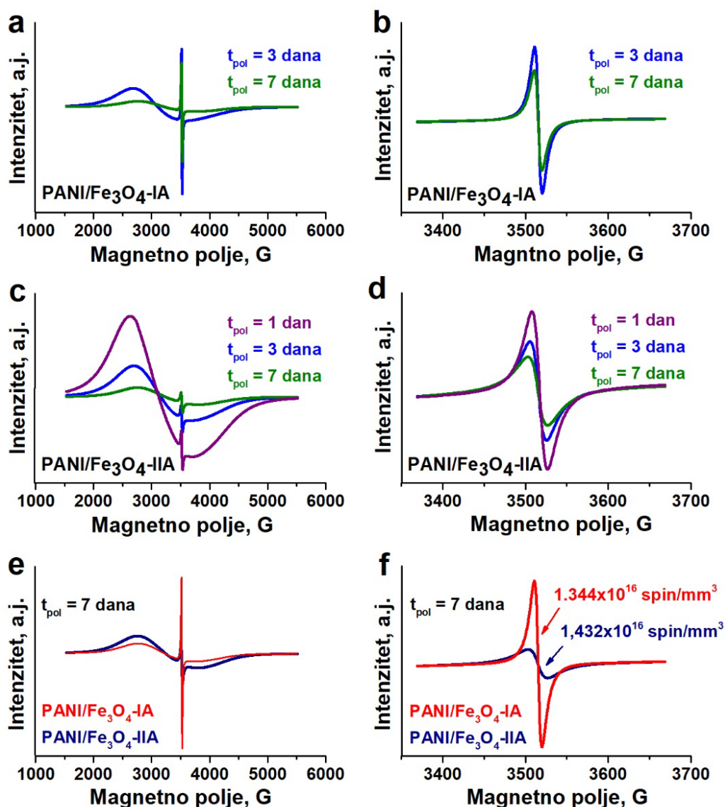
Slika 4.20. (a,b) EPR spektri uzoraka PANI/ \text{Fe}_3\text{O}_4 -IA prikazani u rasponu od 4000 G (a) i 300 G (b); (c,d) EPR spektri uzoraka PANI/ \text{Fe}_3\text{O}_4 -IIA prikazani u rasponu od 4000 G (c) i 300 G (d); (e,f) Poređenje EPR spektara uzoraka PANI/ \text{Fe}_3\text{O}_4 -IA(7) i PANI/ \text{Fe}_3\text{O}_4 -IIA(7) prikazanih u rasponu od 4000 G (e) i 300 G (f).
