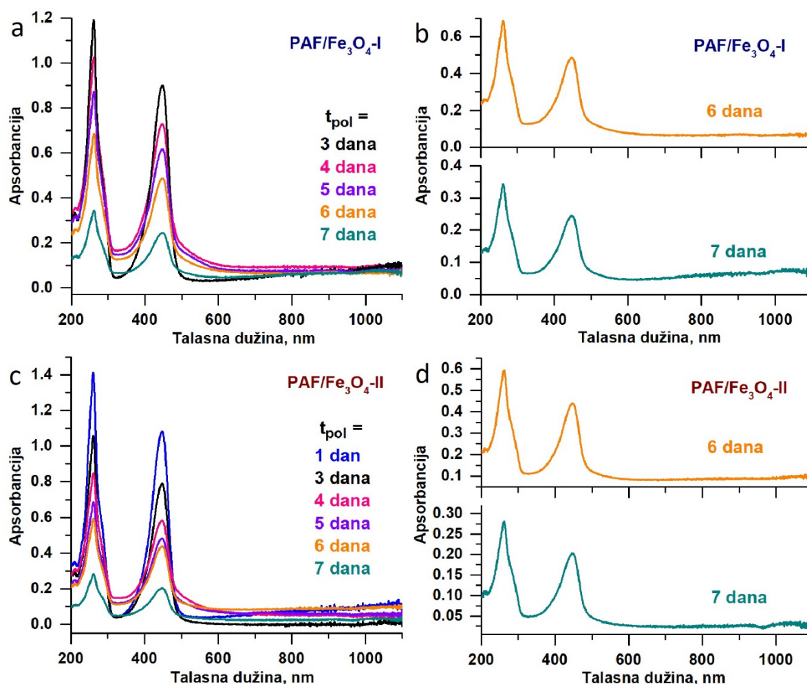
Slika 4.47. UV-Vis-NIR spektri reakcionih suspenzija PAF/Fe 3 O 4 -I (a i b) i PAF/Fe 3 O 4 -II (c i d) razblaženih u vodi 4000 puta.
