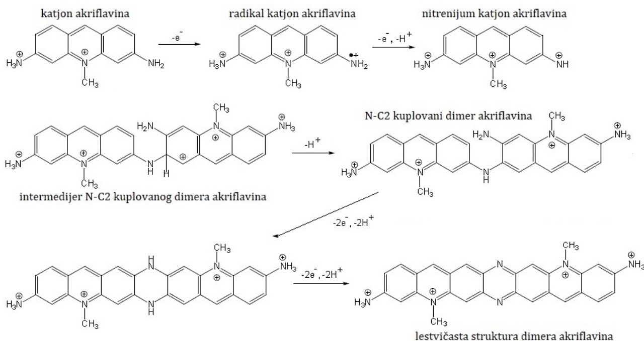
Slika 1.27. Shematski prikaz dimerizacije akriflavina koji odgovara mehanizmu predloženom u radu Synthesis and characterization of polyacriflavine, B. Marjanović, G. Čirić-Marjanović. Radulović, I. Juranić, P. Holler, Materials Science Forum. 555 (2007) 503-508.
