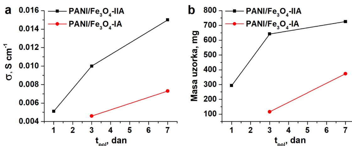
Slika 4.15. Uticaj uslova sinteze ( t_{\text{pol}} i m(\text{Fe}_3\text{O}_4)/m(\text{ani}) ) na (a) električnu provodljivost i (b) masu uzoraka PANI/Fe 3 O 4 -IA i PANI/Fe 3 O 4 -IIA.
