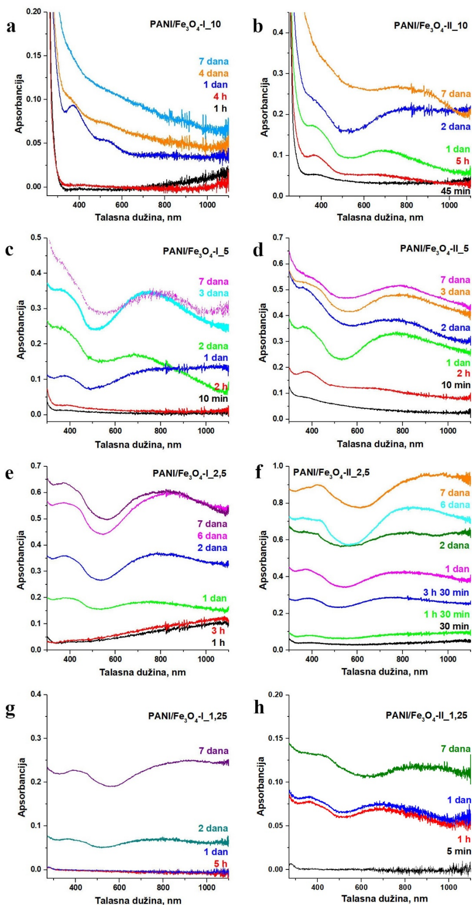
Slika 4.5. UV-Vis-NIR spektri suspenzija reakcionih sistema PANI/Fe 3 O 4 razblaženih u vodi 10 puta.
