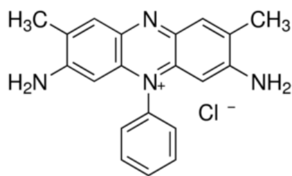
Slika XX. Safranin O.
