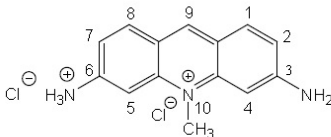
Slika 1.26. Akriflavin hidroklorid.
