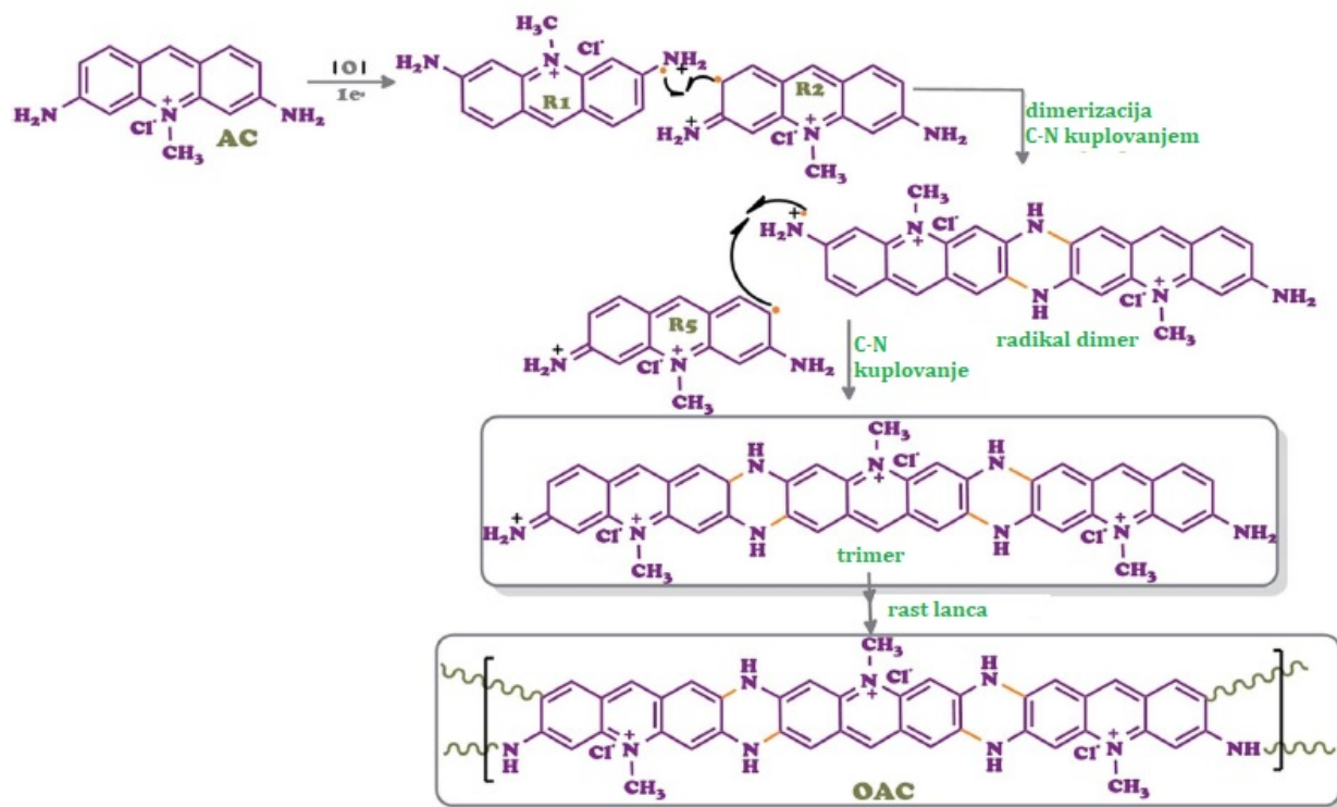
Slika 1.28. Predloženi mehanizam oksidacije akriflavina sa \text{H}_2\text{O}_2 . Slika preuzeta i adaptirana sa dozvolom iz RSC Advances, Synthesis, characterization and photovoltaic studies of oligo(acriflavine) via chemical oxidative polymerization, autora F. Kolcu, I. Kaya, 7, 8973-8984. Copyright (2017) The Royal Society of Chemistry.
