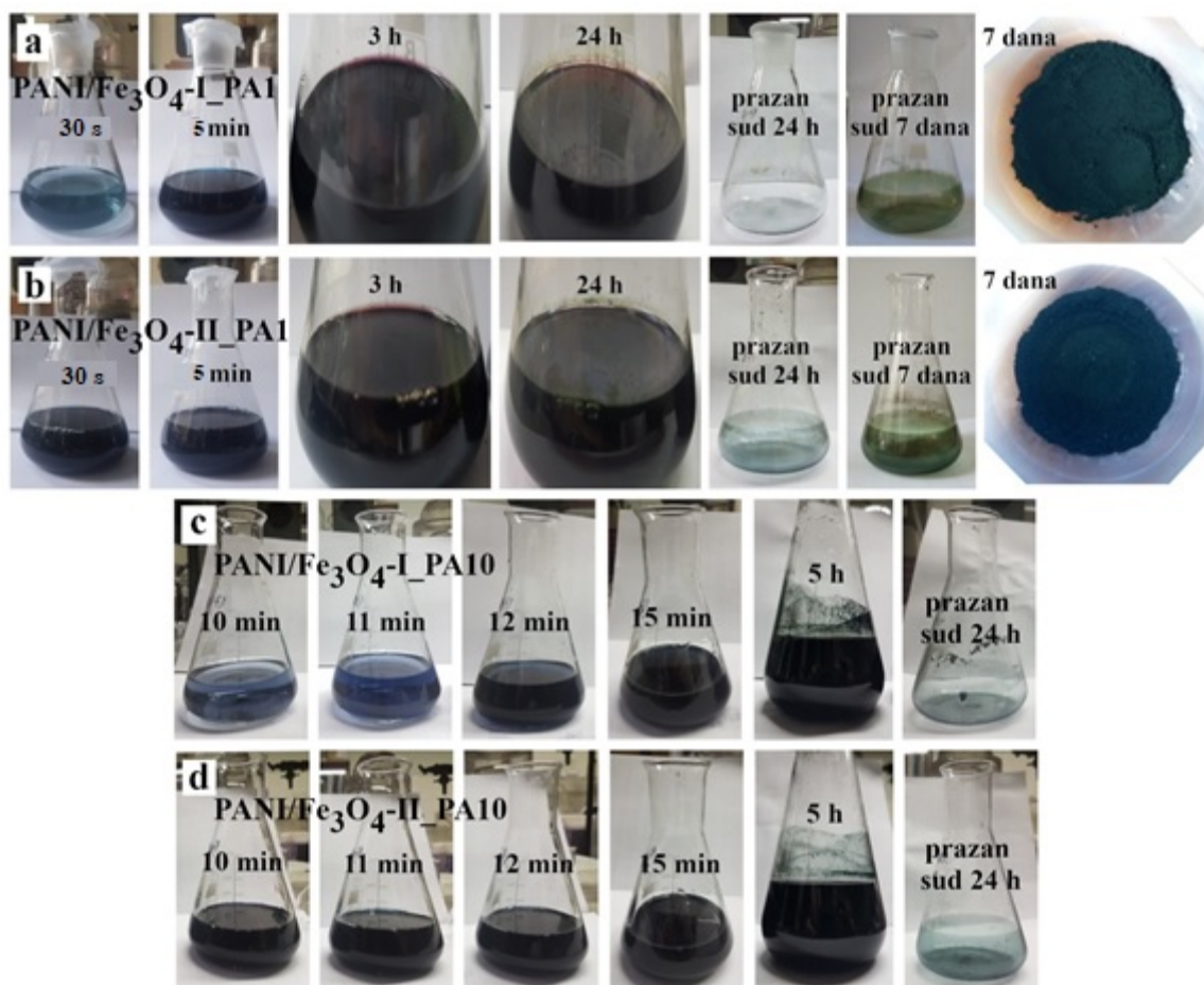
Slika 4.29. Promene boje reakcionih smeša tokom oksidacije anilina u prisustvu p-ADPA sa oksidansom \text{H}_2\text{O}_2 /APS.
