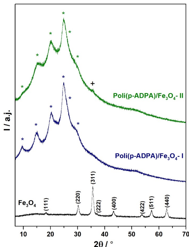
Slika 4.42. Difraktogrami prahova Poly(p-ADPA)/Fe 3 O 4 -I i Poly(p-ADPA)/Fe 3 O 4 -II i nanočestica Fe 3 O 4 .
