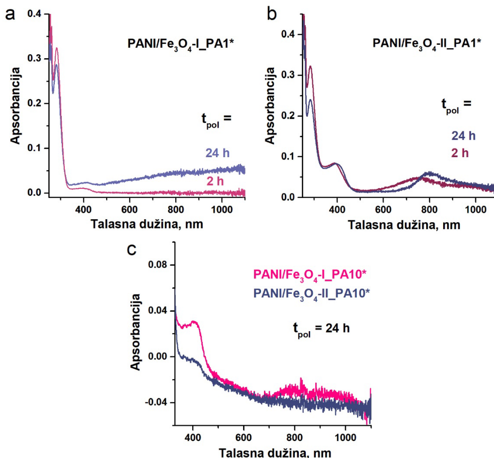
Slika 4.28. UV-Vis-NIR spektri suspenzija reakcionih smeša snimjeni tokom oksidacije anilina u prisustvu p-ADPA bez dodatog oksidansa. Suspenzije PANI/Fe 3 O 4 -I_PA1* i PANI/Fe 3 O 4 -II_PA1* ( a i b ) su neposredno pre merenja razblažene u vodi 10 puta, dok su suspenzije PANI/Fe 3 O 4 -I_PA10* i PANI/Fe 3 O 4 -II_PA10* ( c ) razblažene 45 puta.
