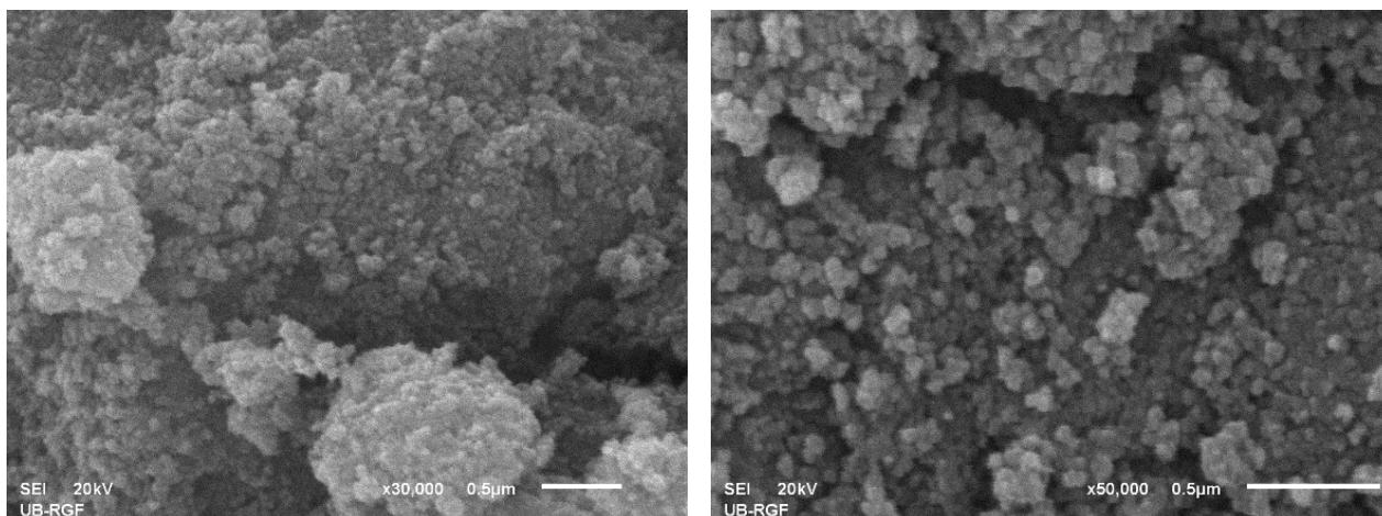
Slika 4.3. SEM mikrografije sintetisanih nanočestica \text{Fe}_3\text{O}_4 pri uvećanjima x30000 (levo) i x50000 (desno).
