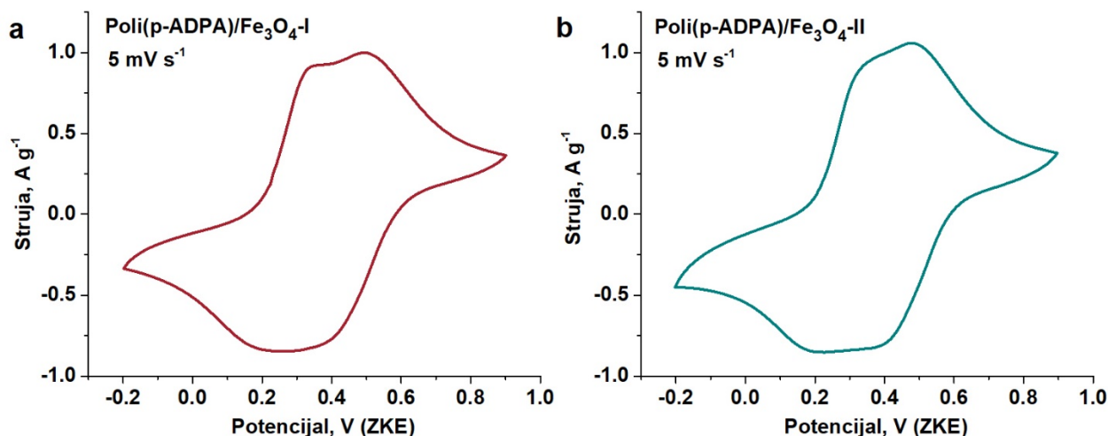
Slika 4.43. Ciklični voltamogrami uzoraka Polip-ADPA/Fe 3 O 4 -I i Polip-ADPA/Fe 3 O 4 -II snimljeni u 1 M HCl pri brzini polarizacije 5 mV·s -1 u opsegu potencijala od -0,2 V do 0,9 V u odnosu na ZKE.
