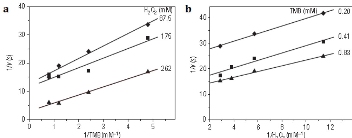
Slika 1.5. Dvostruko recipročni grafici aktivnosti nanočestica \text{Fe}_3\text{O}_4 pri fiksnoj koncentraciji jednog supstrata naspram promenljive koncentracije drugog supstrata za \text{H}_2\text{O}_2 i TMB. Nagib linija je paralelan, što je karakteristično za ping-pong mehanizam. Slika preuzeta i adaptirana sa dozvolom iz Nature Nanotechnology, Intrinsic peroxidase-like activity of ferromagnetic nanoparticles, autora L. Gao, J. Zhuang, L. Nie, J. Zhang, Y. Zhang, N. Gu, T. Wang, J. Feng, D. Yang, S. Perrett, X. Yan, 2, 577–583. Copyright (2007) Nature Publishing Group.
