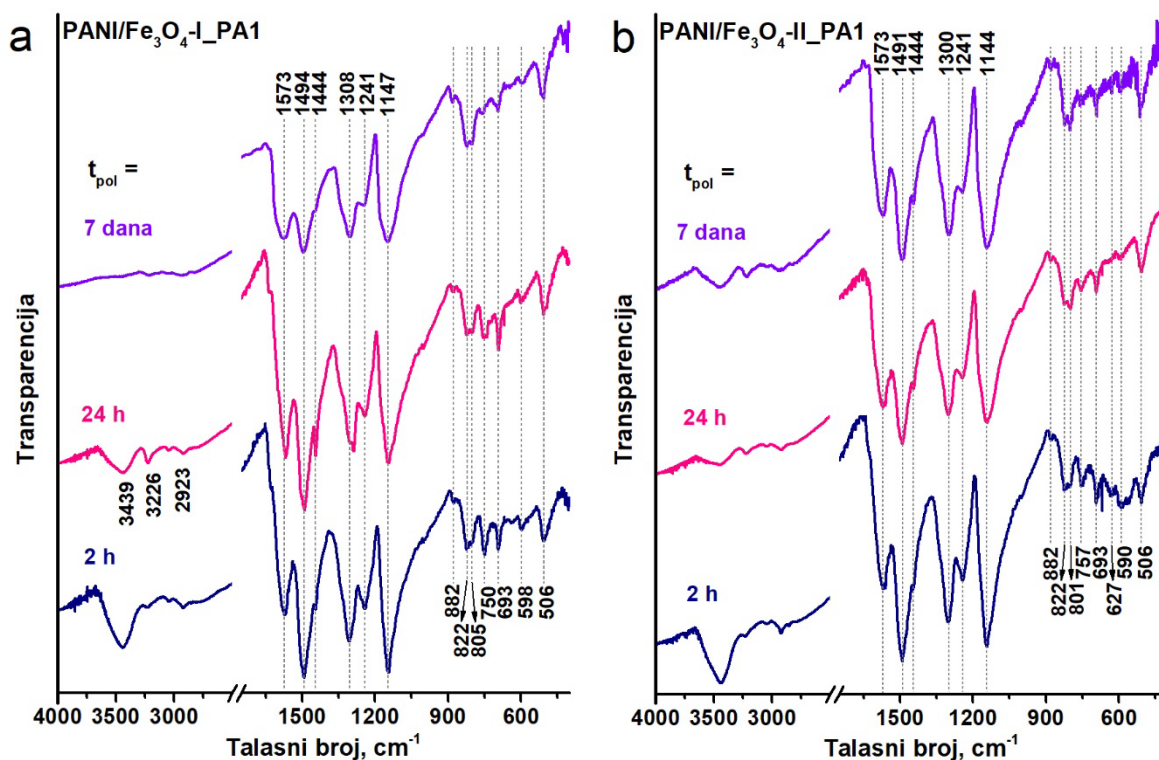
Slika 4.32. FTIR spektri uzoraka PANI/Fe 3 O 4 -I_PA1 ( a ) i PANI/Fe 3 O 4 -II_PA1 ( b ).
