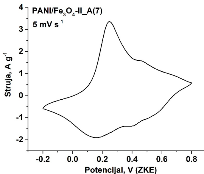
Slika 4.22. Ciklični voltamogram PANI/Fe 3 O 4 -II_A(7) snimljen u 1 M HCl pri brzini polarizacije 5 \text{ mV} \cdot \text{s}^{-1} u opsegu potencijala od -0,2 V do 0,8 V u odnosu na ZKE.
