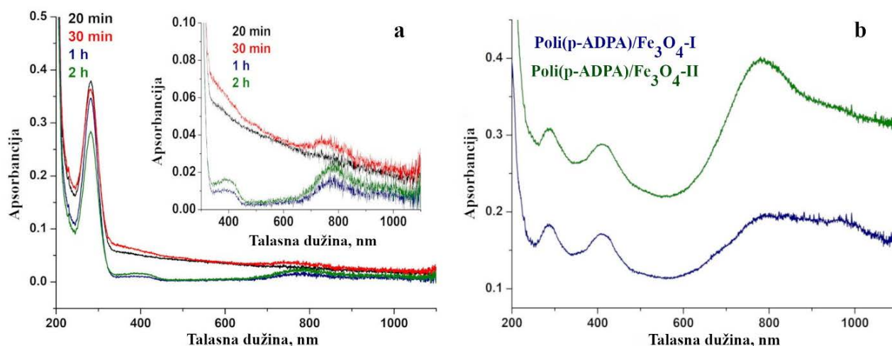
Slika 4.37. UV-Vis-NIR spektri (a) suspenzija kontrolne reakcije (bez nanočestica \text{Fe}_3\text{O}_4 ) razblaženih u vodi 100 puta (umetnuta slika prikazuje deo spektra u oblasti 300-1100 nm); (b) suspenzija praškastih uzoraka Poli(p-ADPA)/ \text{Fe}_3\text{O}_4 -I i Poli(p-ADPA)/ \text{Fe}_3\text{O}_4 -II u 0,1 M HCl (uzorci sintetisani za t_{\text{pol}} = 2 h) [267].
