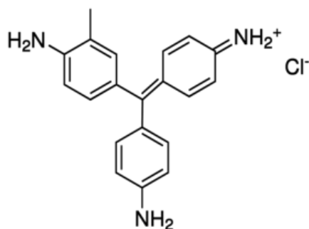
Slika 1.30. Fuksin bazni.
