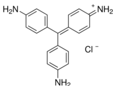
Slika 1.29. Pararozanilin hidrohlorid.
