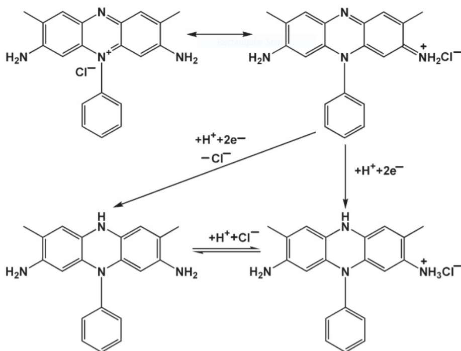
Slika 1.31. Predloženi mehanizam elektrohemijskih redoks reakcija safranina. Slika preuzeta i adaptirana sa dozvolom iz Thin Solid Films, Electrosynthesis and characterisation of poly(safranine T) electroactive polymer films, autora R. Pauliukaite, A. Selskiene, A. Malinauskas, C.M.A. Brett. 517, 5435–5441. Copyright (2009) Elsevier.
