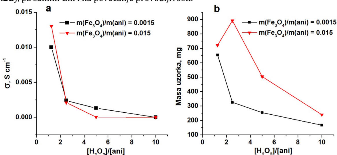
Slika 4.6. Uticaj uslova sinteze (molskog odnosa [H 2 O 2 ]/[ani] i m(Fe 3 O 4 )/m(ani)) na električnu provodljivost ( a ) i masu ( b ) uzoraka PANI/Fe 3 O 4 .
