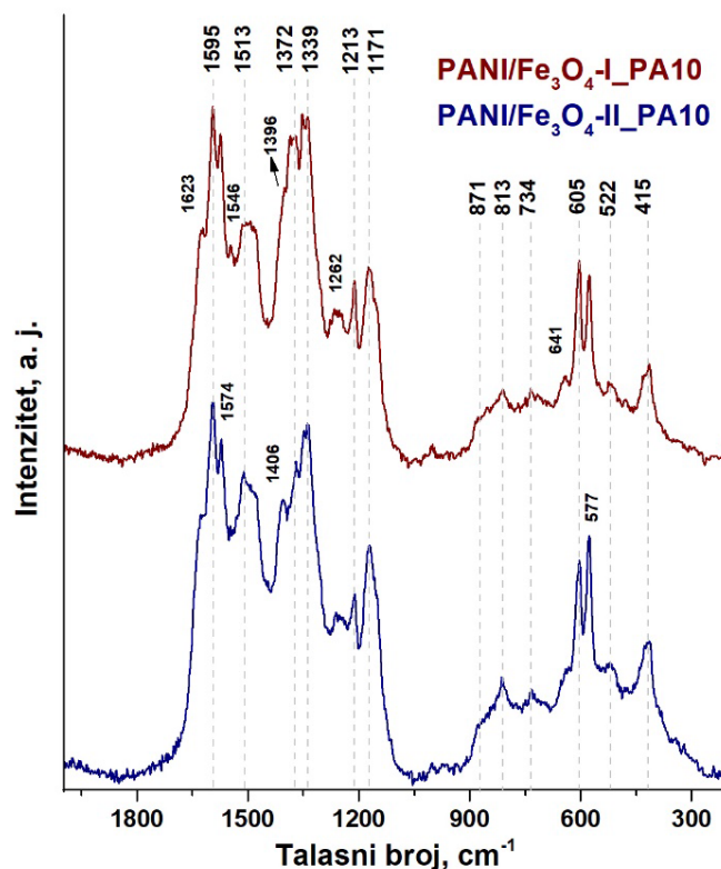
Slika 4.35. Ramanski spektri uzoraka PANI/Fe 3 O 4 -I_PA10 i PANI/Fe 3 O 4 -II_PA10.
