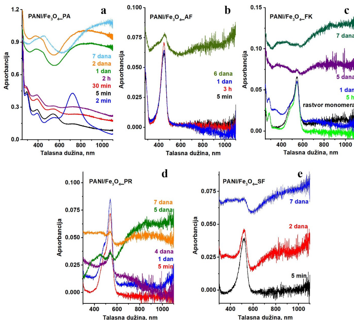
Slika 4.24. UV-Vis-NIR spektri razblaženih suspenzija reakcionih smeša tokom oksidacije anilina sa \text{H}_2\text{O}_2/\text{APS} u prisustvu različitih arilamina. Suspenzije razblažene u vodi 100 puta.
