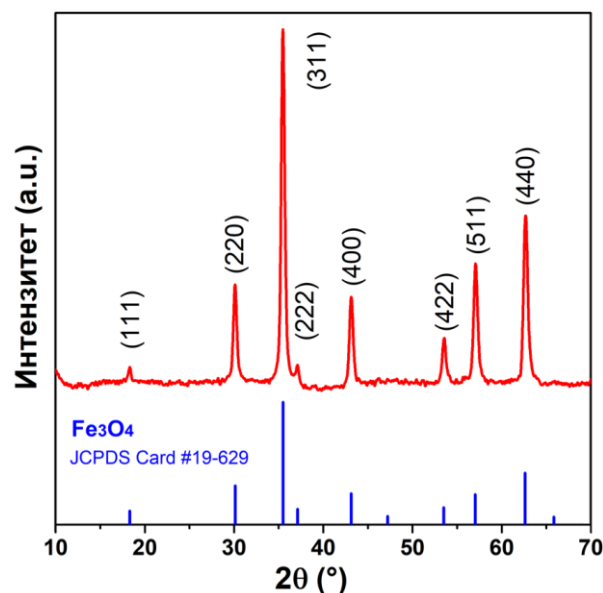
Слика 5.22. Дифрактограм синтетисаних IONPs ( goFe ) и симулирани дифрактограм за Fe 3 O 4 (JCPDS #19-629) ( доле ).
