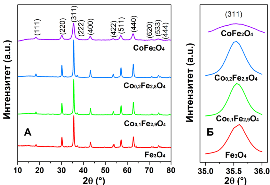
Слика 5.6. (А) Дифрактограми \text{Co}_x\text{Fe}_{3-x}\text{O}_4 наночестица и (Б) постепено померање положаја (311) рефлексije при промени концентрације кобалта.
