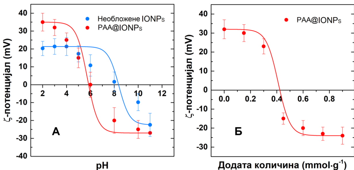
Слика 5.23. (А) Зависност зета потенцијала од рН за необложене IONPs и PAA@IONPs и (Б) Зависност зета потенцијала од количине PAA током поступка облагања наночестица на рН 6,5. Криве зета потенцијала показују облик Boltzmann -ове сигмоидне функције.
