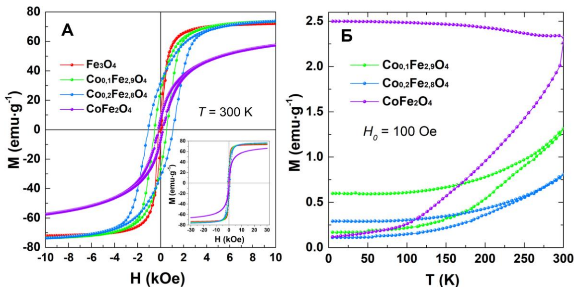
Слика 5.10. (А) Магнетизација у зависности од јачине поља на 300 К у областима ниских поља и (Б) Зависност магнетизације од температуре у ZFC/FC режиму мерења. Уметнута слика на 5.10А је M = f(H) крива у областима високих поља.
