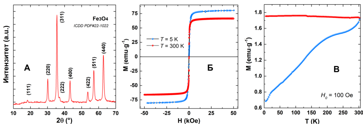
Слика 5.17. (А) Дифрактограм синтетисаних IONP_A ; (Б) Хистерезисне криве на 5 К и 300 К и (В) Зависност магнетизације IONP_A од температуре у ZFC/FC режиму.
